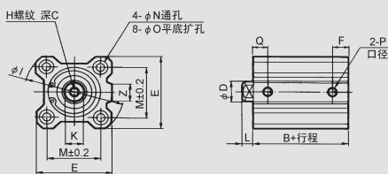
CQ2BΦ12 ~ Φ25
